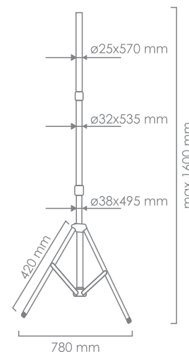
Floodlight stand / Стойка за прожектор 631AD00000040
