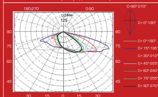
Light Distribution Curve Светлоразпределителна крива
