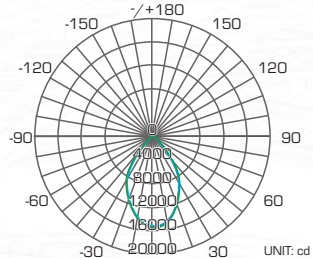
Light Distribution Curve Светлоразпределителна крива
