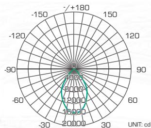
Light Distribution Curve Светлоразпределителна крива
