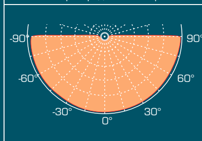
Light Distribution Curve Светлоразпределителна крива
