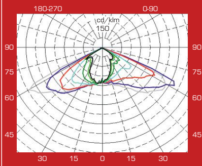
Light Distribution Curve Светлоразпределителна крива
