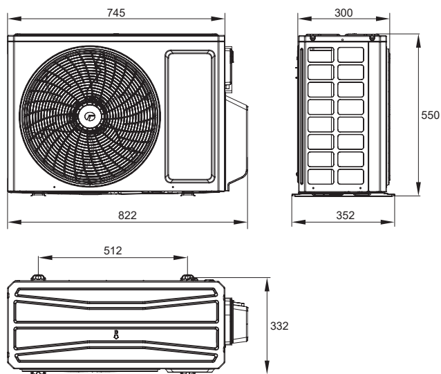
■ GWHD(18)NK600(LC)(LH)
