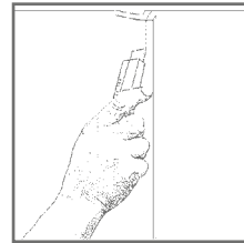
Attaccare il successivo pannello di Climapron Plus in modo ermetico sul giunto oppure sovrapponendolo al precedente e tagliando l'eccesso. Per tagliare il Climapron Plus utilizzare un cutter.
